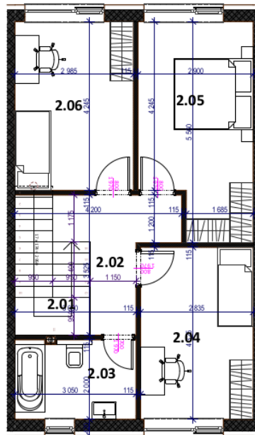
PÔDORYS POSCHODIA
