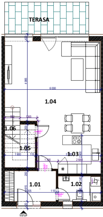
PÔDORYS PRÍZEMIA
