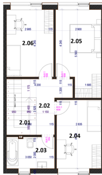
PÔDORYS POSCHODIA
